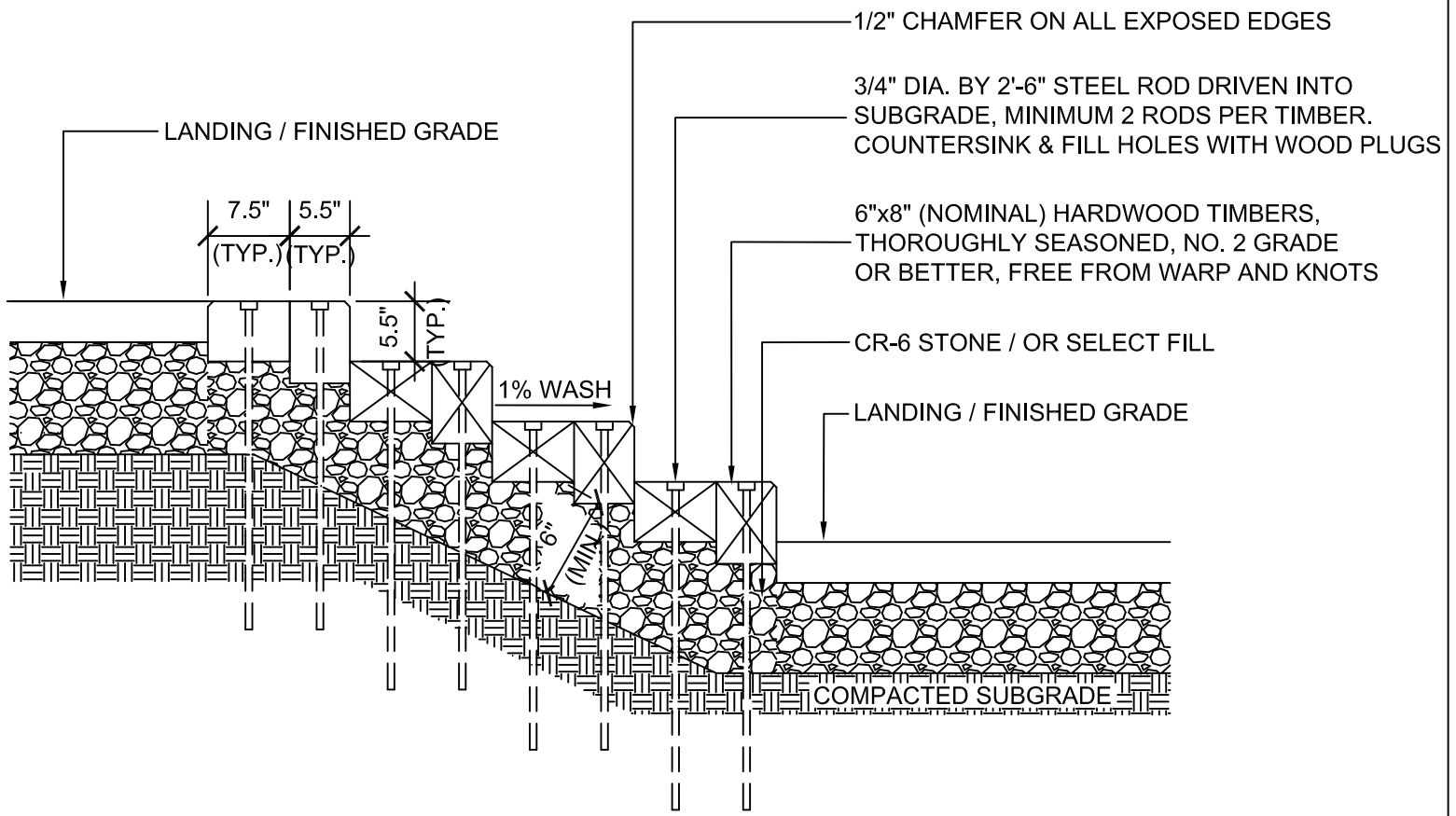
SECTION N.T.S.
