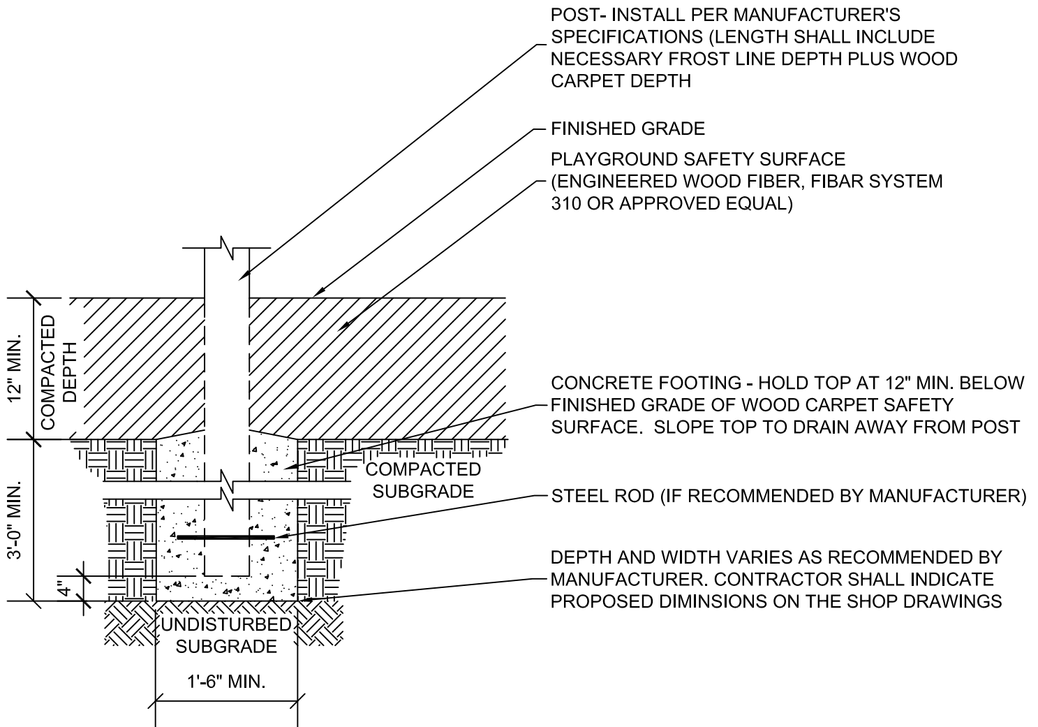
SECTION N.T.S.
