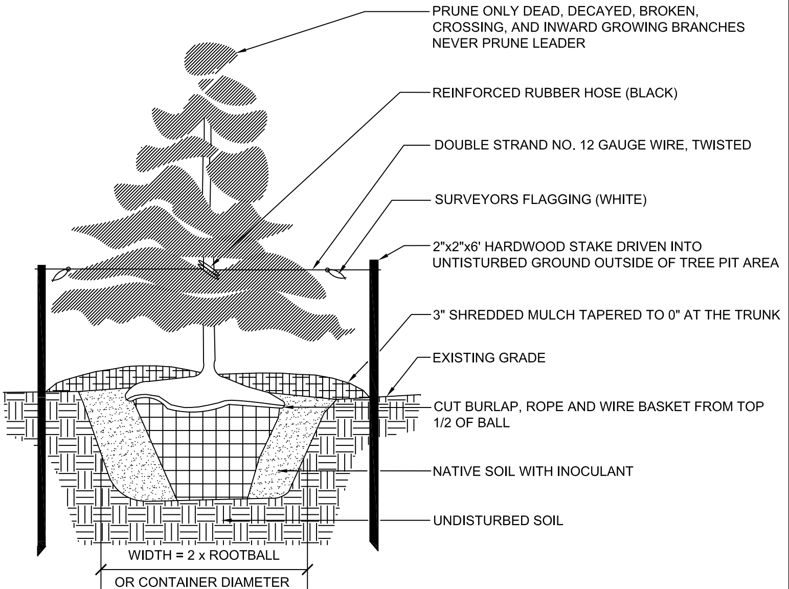
SECTION N.T.S.
