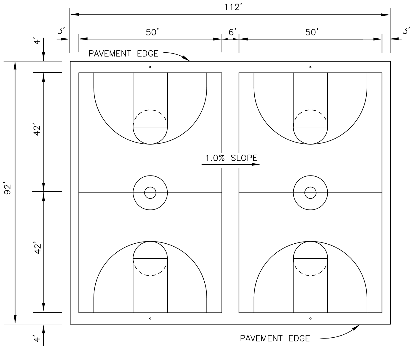
PLAN N.T.S.
