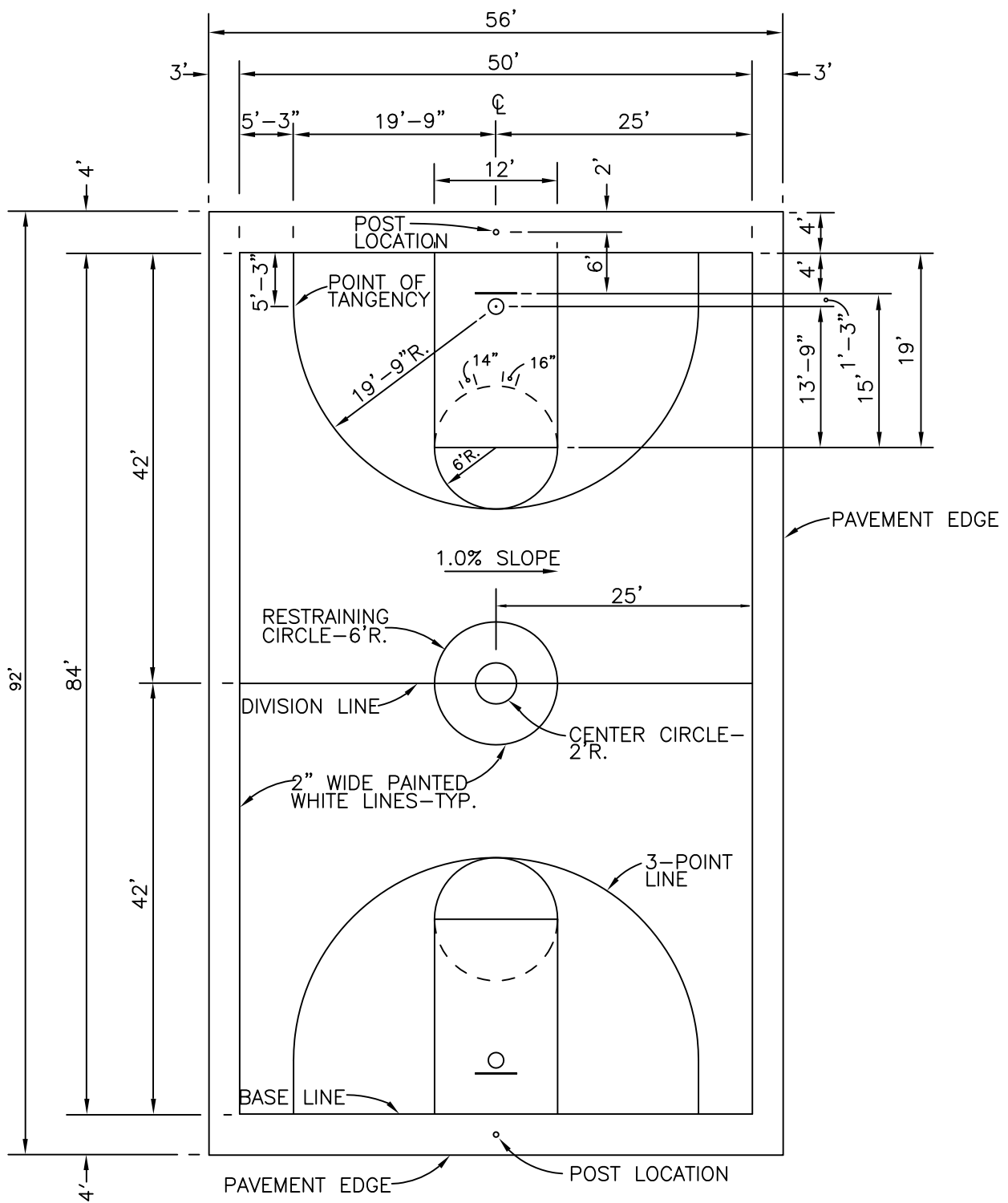
PLAN N.T.S.
