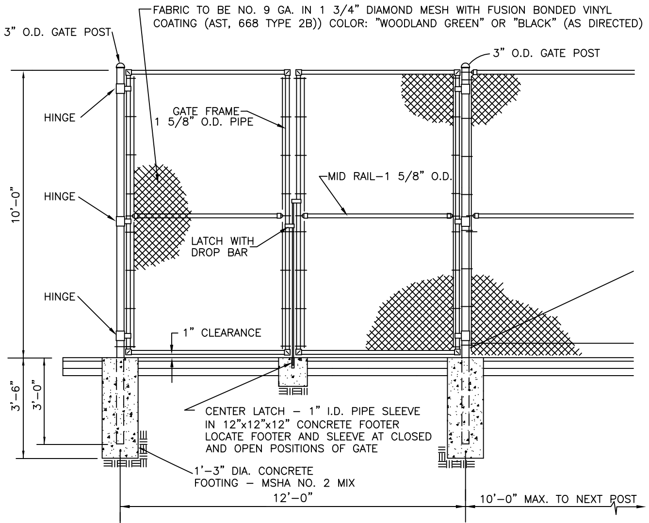
ELEVATION N.T.S.
