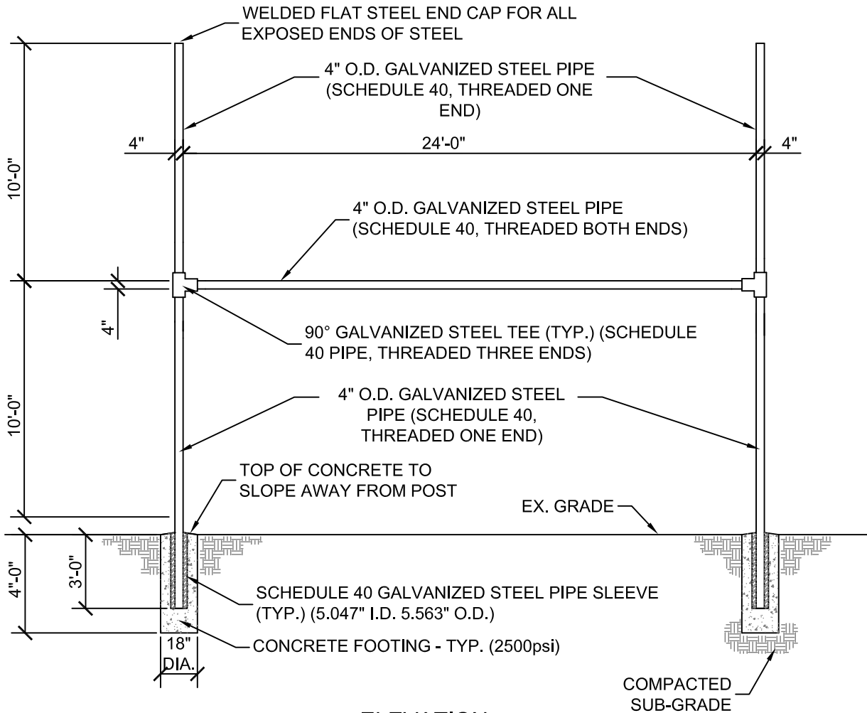
ELEVATION N.T.S.
