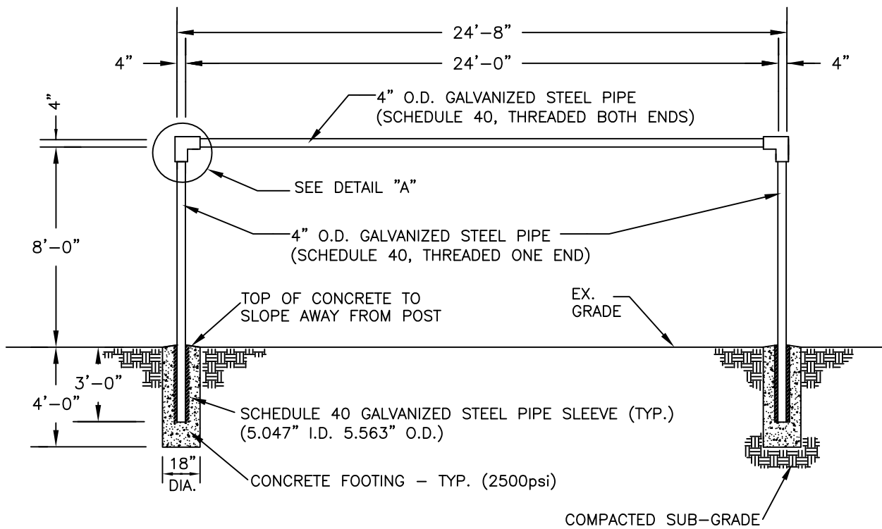
ELEVATION N.T.S.
