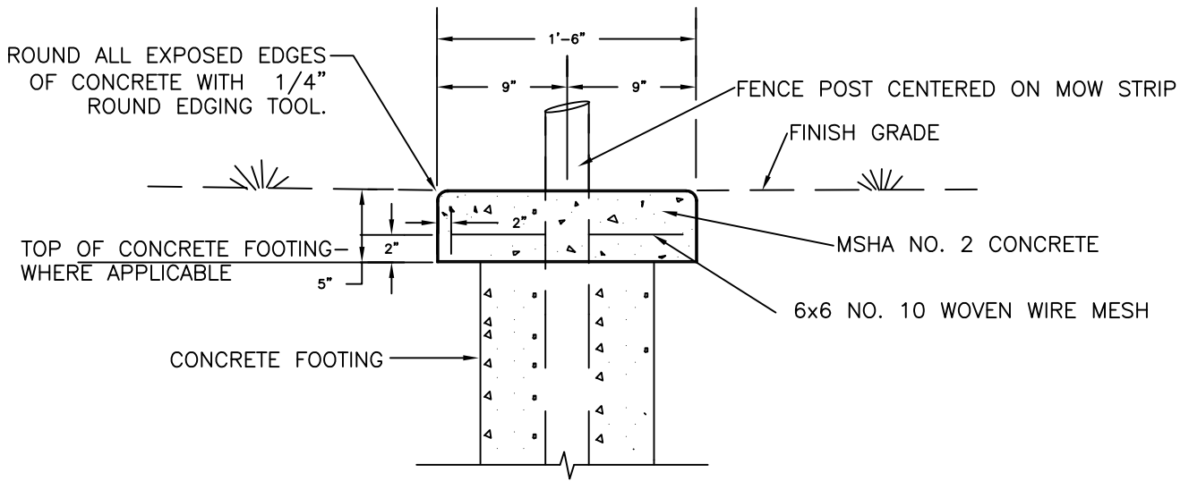
SECTION N.T.S.
